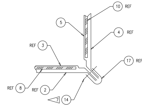
SECTION G-G SCALE: 2/1 2X
